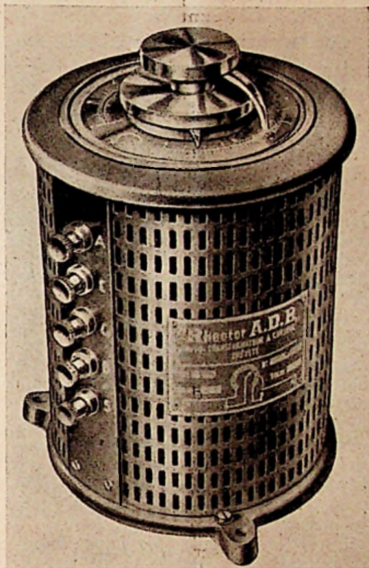
1 Phase transformator met 2 regelkringen
